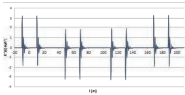
4. Wykresy przyspieszeń ruchu drgającego \ddot{X}(l) dla Przypadku 5 (odcinki krzywizny liniowej, k_1 = k_3 = 0 )
