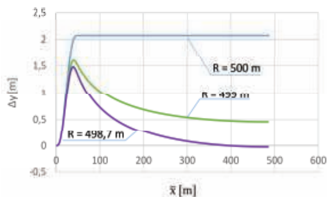
9. Wykresy różnic rzędnych na długości zmodyfikowanego układu geometrycznego dla R = 500 m, 499 m i 498,7 m, l_k = 70 m, l_w = 120 m ( \alpha = 135^\circ )
