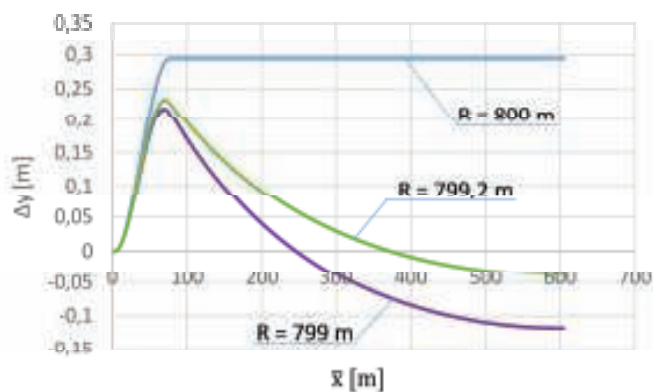
7. Wykresy różnic rzędnych na długości zmodyfikowanego układu geometrycznego dla R = 800 m, 799 m i 799,2 m, l_k = 90 m, l_w = 110 m ( \alpha = 90^\circ )
