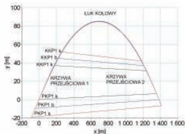
5. Układ łuku kołowego z dwiema krzywymi przejściowymi przedstawiony w trzech wariantach: z zastosowaniem klotoidy, krzywej Blossa i sinusoidy
